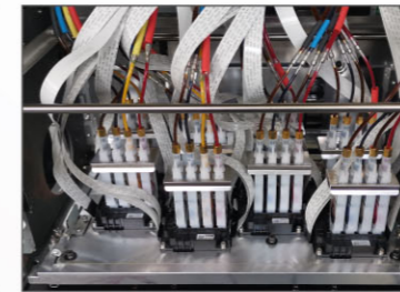
Печатающие головки
